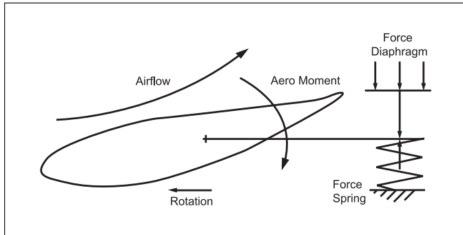
AV Force Diagram Fig. 16
