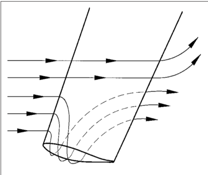
Tip Vortex (Leakage) Fig. 5
